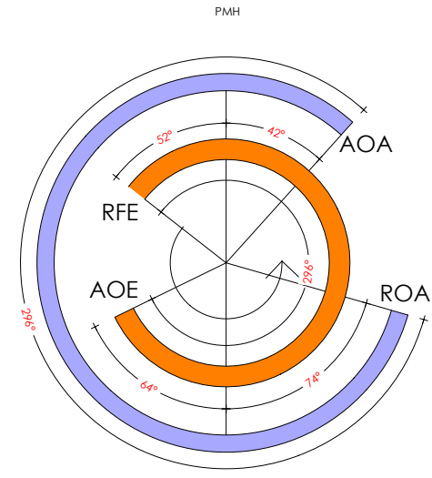
Laverda 750 SF
