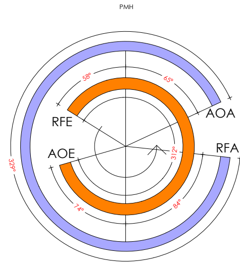
Ducati 750 GT
