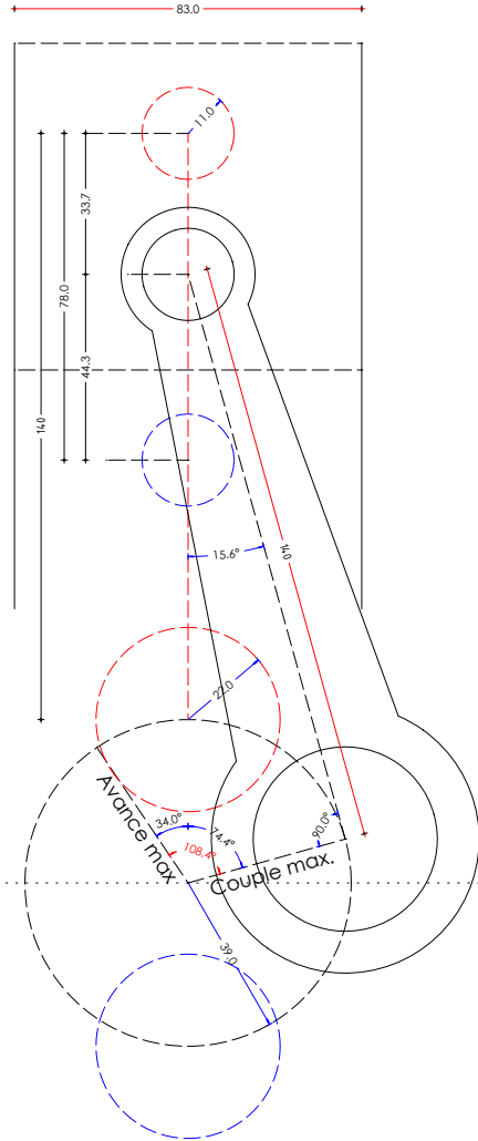
Guzzi 850 le Mans II Al x c: 83x78 Bielle courte 140 (<2x78) Rapport vol: 10:1
