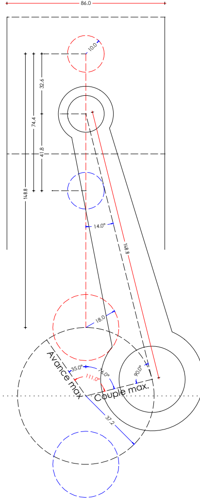
Ducati 850 gt Al x c: 86x74.4 Bielle moyenne 148.8 (=2x74.4) Rapport vol: 9:1
